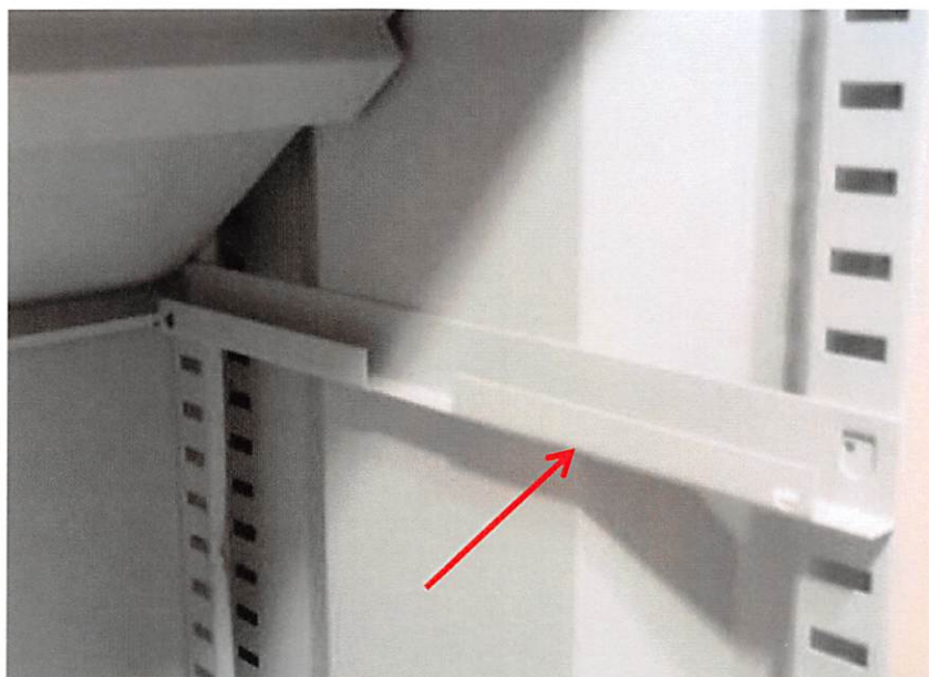
Situação existente. Reaproveitar cantoneira em formato "L" para apoiar os perfis metálicos.
