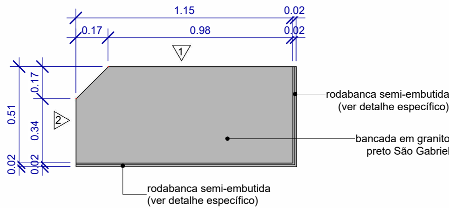
Bancada 02 - Vista Superior
