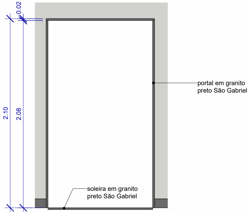
4 CORTE CC PORTAL E SOLEIRA 1 : 25
