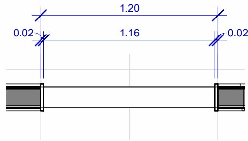
3 COPAS - PLANTA BAIXA PORTAL E SOLEIRA 1 : 25
