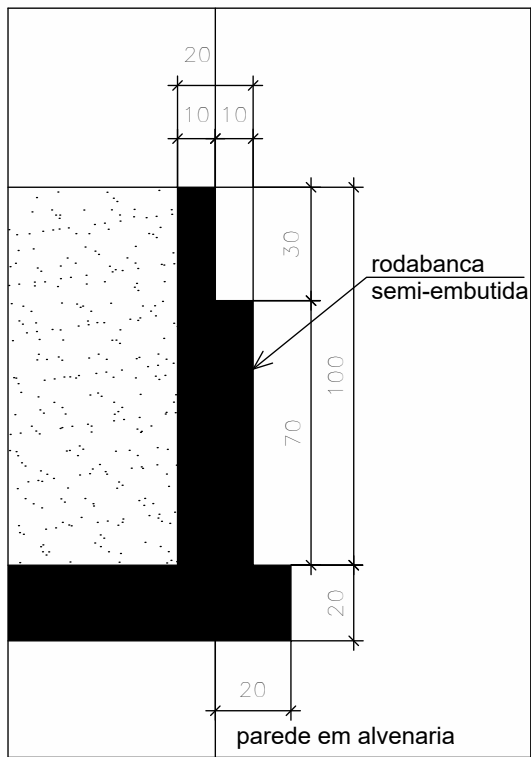
DET. RODABANCADA - VISTA LATERAL 1 : 2
