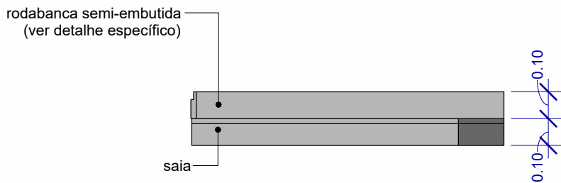
Bancada 02 - Elevação 01
