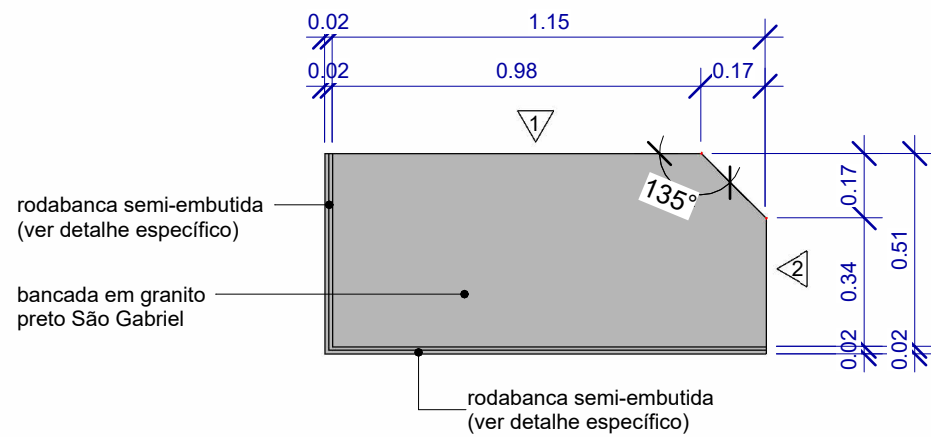
Bancada 01 - Vista Superior
