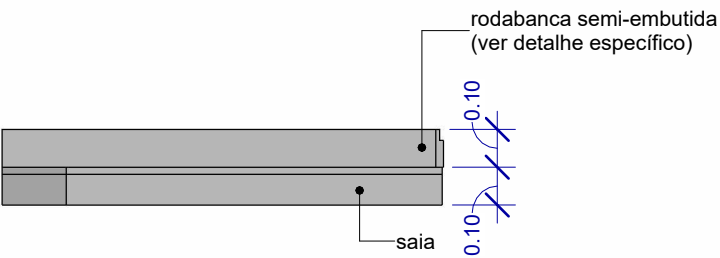
Bancada 01 - Elevação 01
