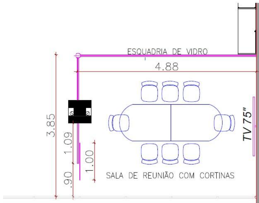
Figura 2 - Croqui de detalhe da sala com divisórias em vidro e porta de correr.
